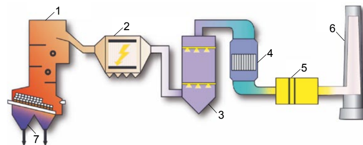
1 – katilas; 2 – elektrostatinis filtras; 3 – skruberis; 4 – azoto oksidų katalizatorius; 5 – sunkiųjų metalų ir dioksinų katalizatorius; 6 – kaminas; 7 – pelenų ir šlakų šalinimas.
